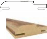
En: 10 / 12 / 14 / 16 / 18 / 20 / 22 cm Boy: 210 cm Kalınlık: 3,6 cm
