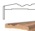
En: 18 / 10 cm Tırnak Uzunluğu: 3 / 4,3 cm Boy: 220 cm
