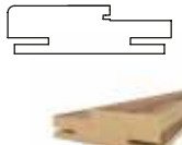
En: 10 / 12 / 14 / 16 / 18 / 20 / 22 cm Boy: 210 cm Kalınlık: 3,6 cm
